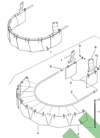
ETB-015810, Ograniczenie szerokości rozsiewu
