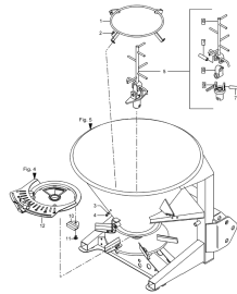
ETB-015809, Pręt mieszadła
