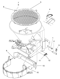
ETB-015808, Rama i zbiornik
