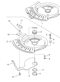
ETB-015811, Dno z otworami
