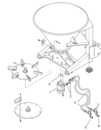
ETB-015813, Napęd hydrauliczny
