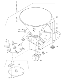
ETB-015812, Rama i zbiornik, tarcze rozsiewające i przekładnia
